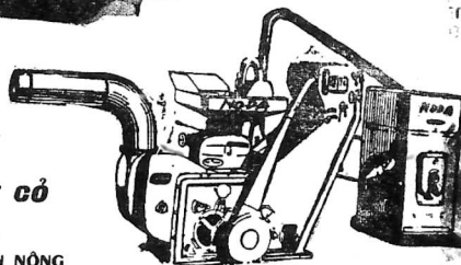
LOẠI DC — CÓ THÙNG NƯỚC VÀ QUẠT GIÓ GIÁ PHÓNG ĐỊNH
