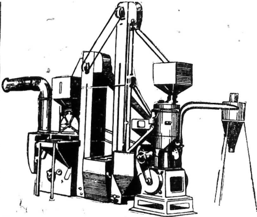
Máy xay lúa loại trung kiểu KRS - 5/KRS - 10 Xay và Chà 500/1000Kg gạo một giờ Giá phỏng định { KRS-5 VNĐ: 440.978 KRS-10 VNĐ: 719.722
