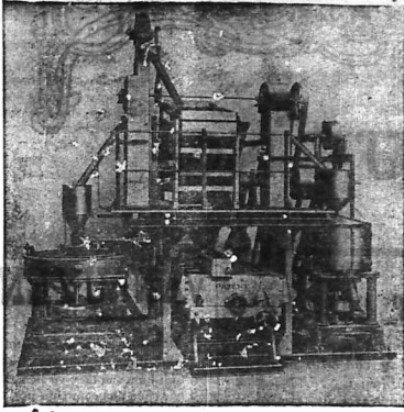
Décortiqueur « FILIPINA » 10 tonnes 1 cône
