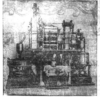
Décortiqueur « FILIPINA » 10 tonnes 1 cône
