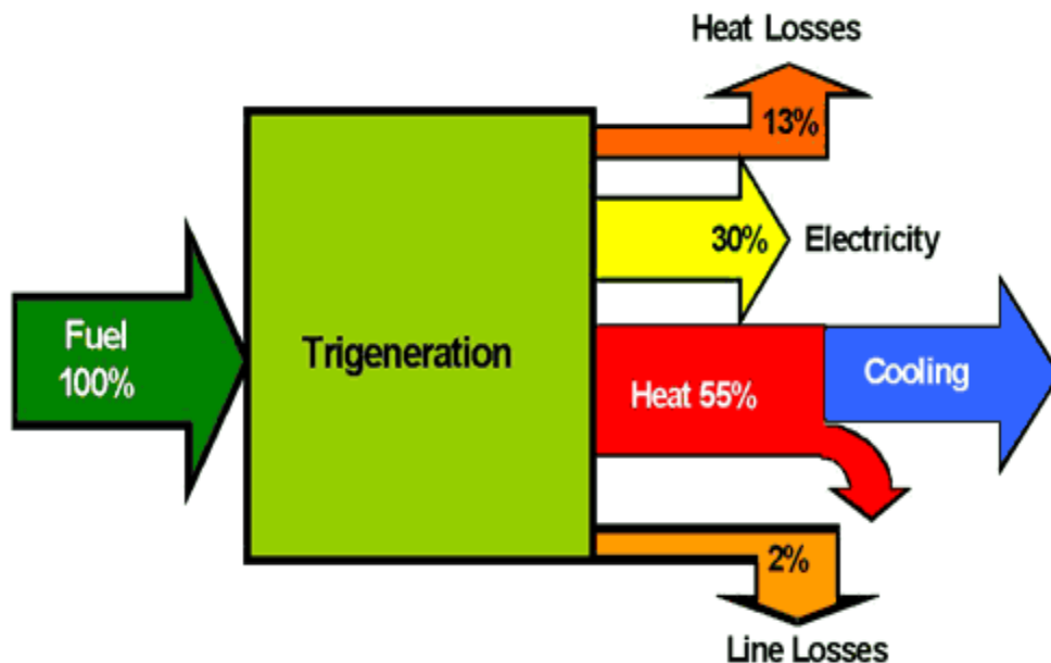
Hệ thống tam phát/trigeneration điển hình gồm một máy chính có thể cùng lúc phát điện, nhiệt lực và nước lạnh.
