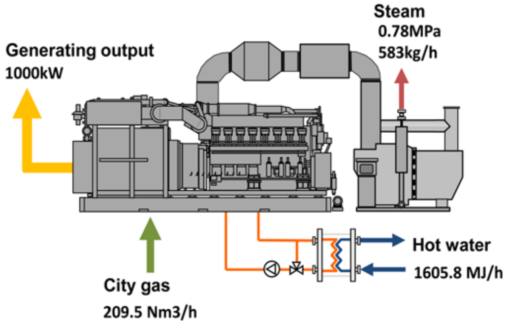
Hệ Thống Cogen tiêu biểu được dùng trong bệnh viện
