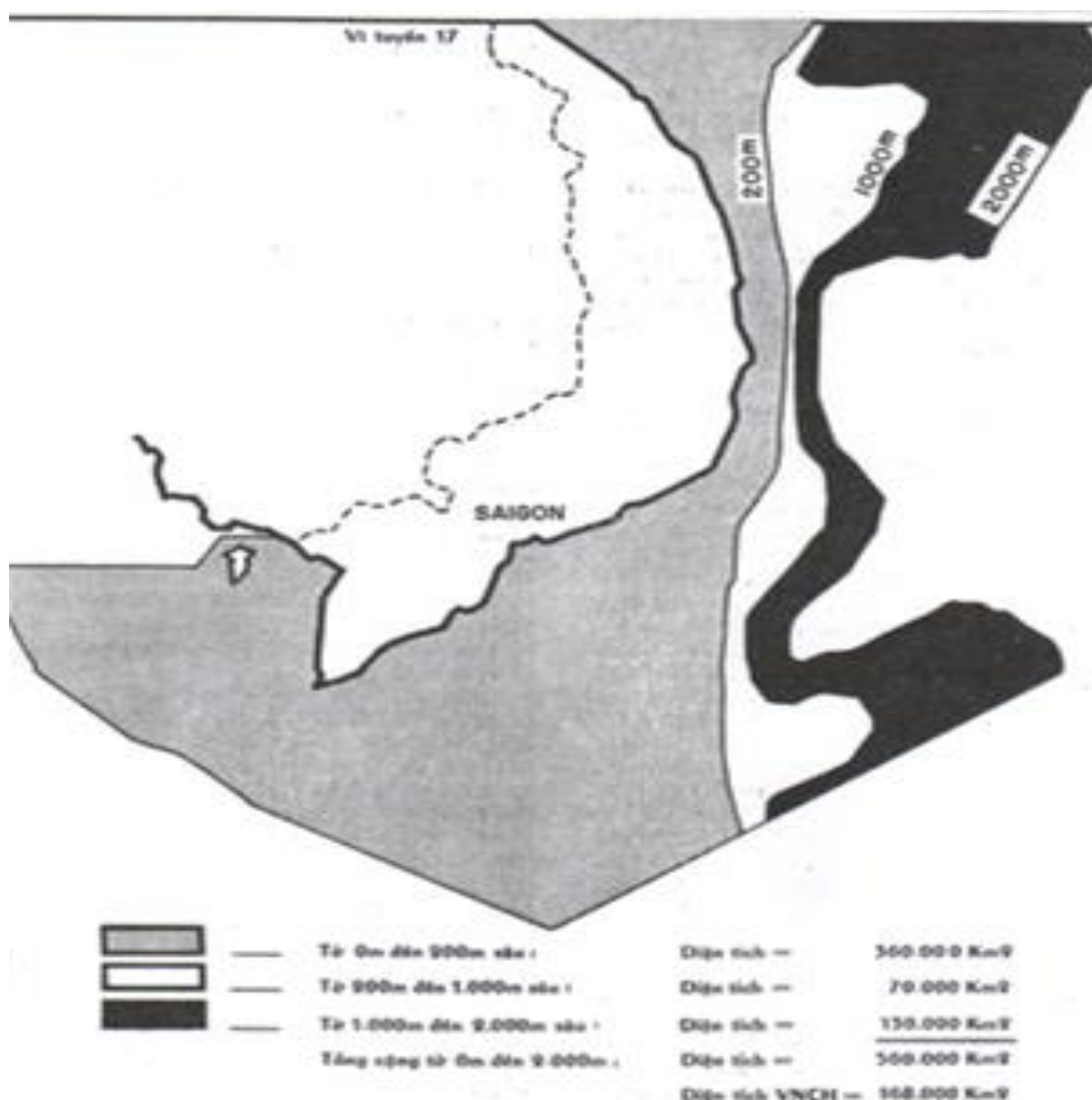
Chiều sâu đo bằng mét của thềm lục địa Việt Nam
